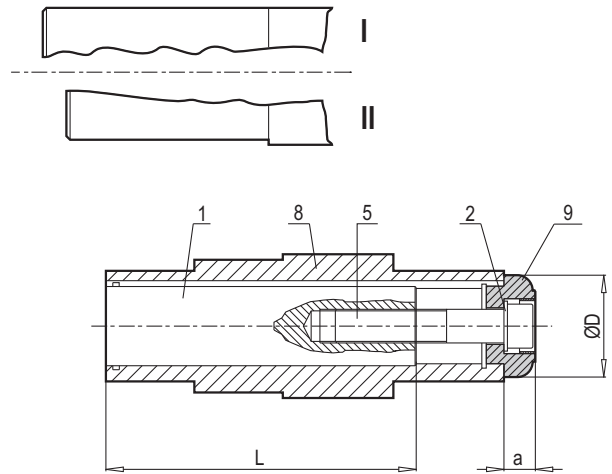
L= Lunghezza massima dell' albero sporgente L= Longueur max. de l'arbre à entraîner L= Longitud máxima del eje macizo
